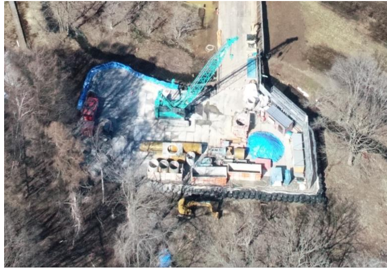
渡島トンネル(台場山) トンネル掘削状況
