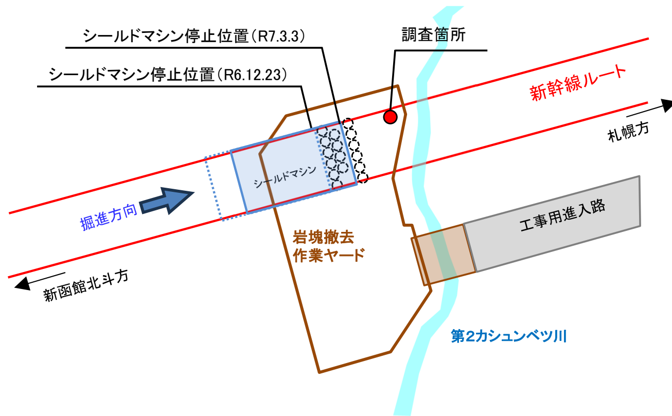
岩塊撤去範囲(区間A①)平面図
