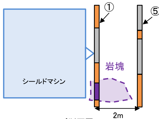
B-B'断面図
